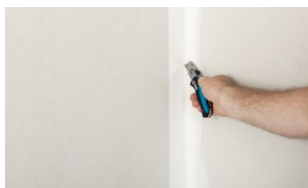
7. Po zaschnutí a přebroušení v rohu odřízněte zbytek pásky Trenn-Fix
