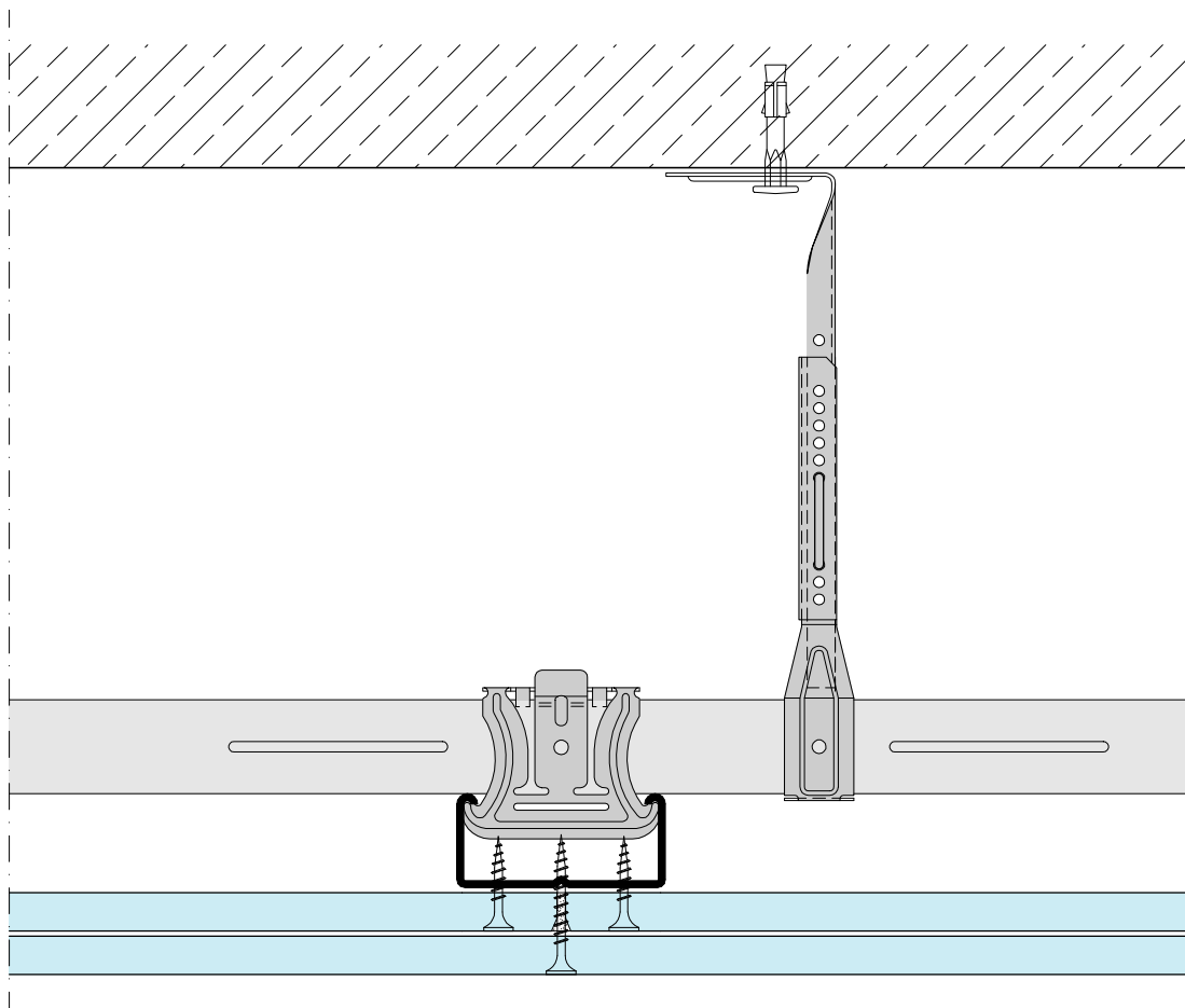
kNAUF D112.cz-C1 Styk řezaných hran - Nosný a montážní profil - třmen noniusový CD
