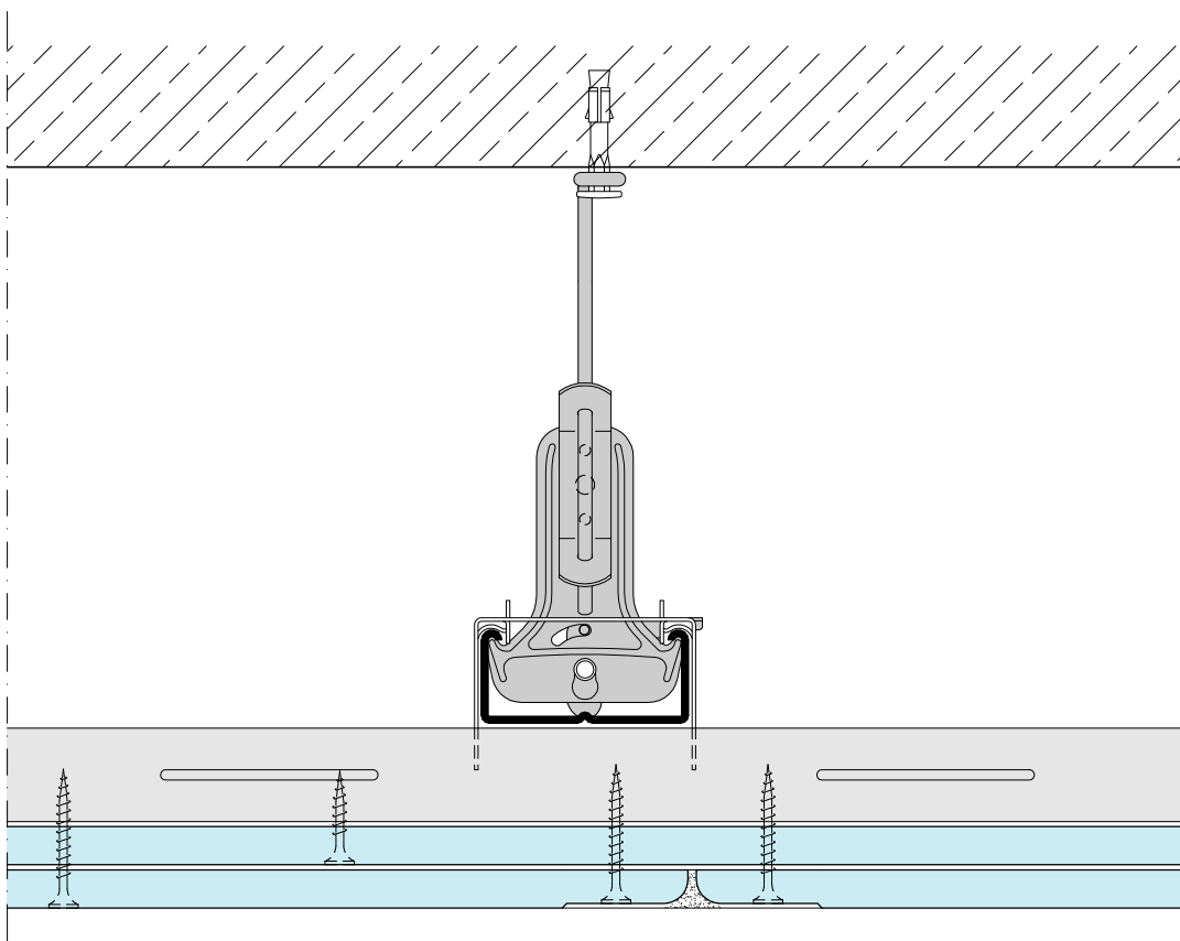
KNAUF D112.cz-B4 Styk podélných hran - Nosný a montážní profil - rychlozávěs s drátem
