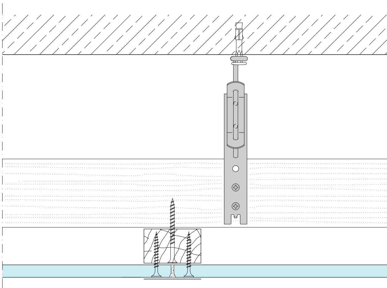
KNAUF D111.cz-C4 Styk řezaných hran - nosná a montážní lať - rychlozávěs
