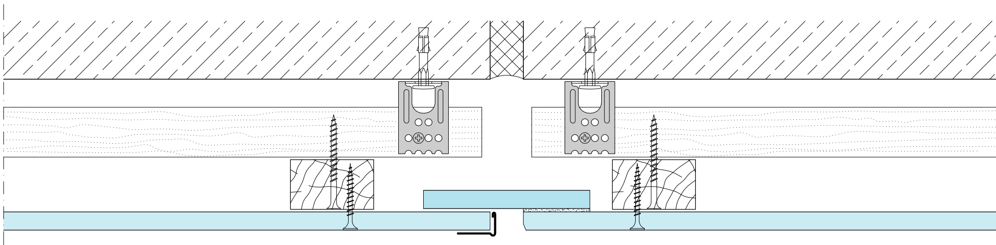
KNAUF D111.cz-C3 Dilatační spára
